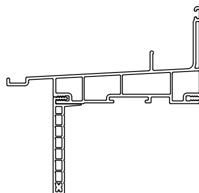
2" FLUSH FIN
