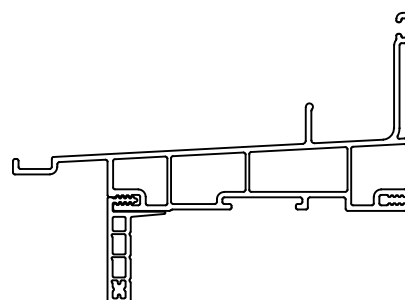
1" FLUSH FIN
